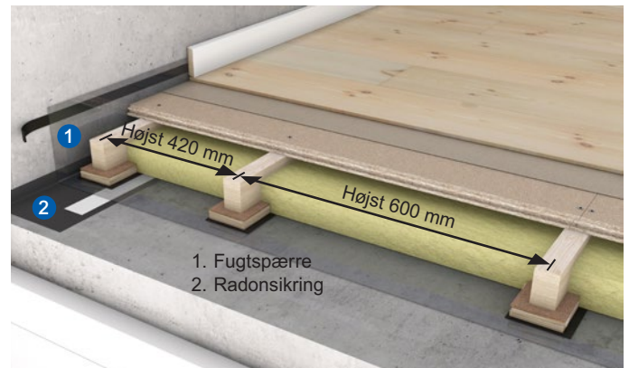
Figur 1 Undergulve på terrændæk bør altid udføres med en fugtspærre og radonspærre på betonoverfladen.
