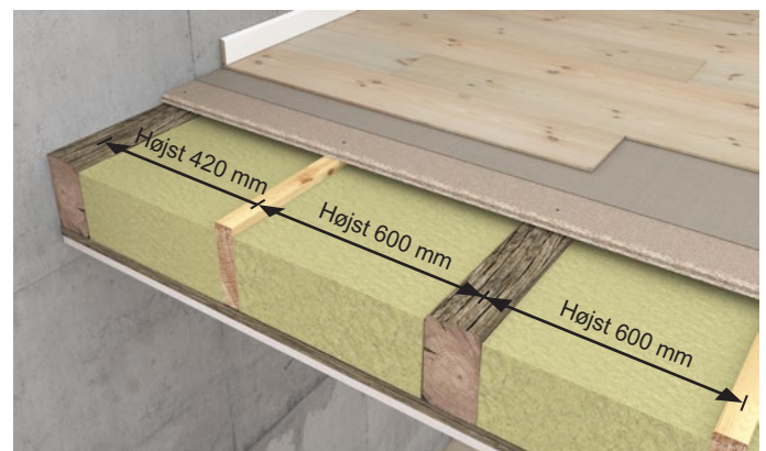
Figur 2 Ældre etagedæk udført med en ekstra bjælke mellem de eksisterende gulvbjælker for at reducere spændvidden til højst 600 mm. Alternativt kan bjælkelaget forstærkes, se Faktablad #1 Forstærkning af ældre bjælkelag på kronospan-dk.dk.
