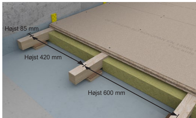
Figur 3 Undergulve lægges med kantstrø højst 85 mm c-c langs alle vægge. Strø- og opklodningsafstande fremgår af tabel 1.
