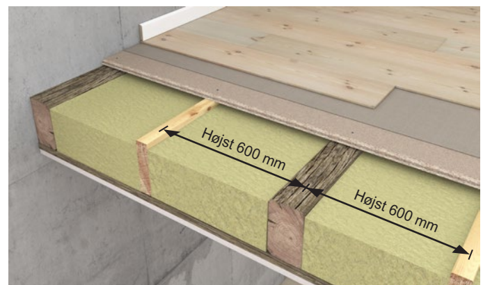
Figur 2 Ældre etagedæk udført med en ekstra bjælke mellem de eksisterende gulvbjælker for at reducere spændvidden til højst 600 mm. Alternativt kan bjælkelaget forstærkes, se Faktblad #1 Forstærkning af ældre bjælkelag på kronospan-dk.dk.
